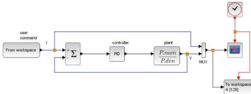
Рис. 1. Приклад моделі у Scilab Xcos
